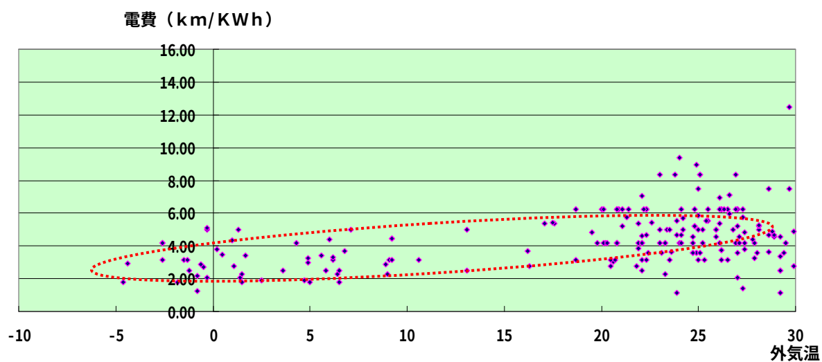
図 5.18 外気温別電費（エアコン有）
