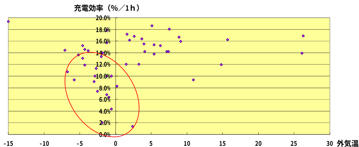
図 5.20 外気温別充電効率散布図 (一般充電)
