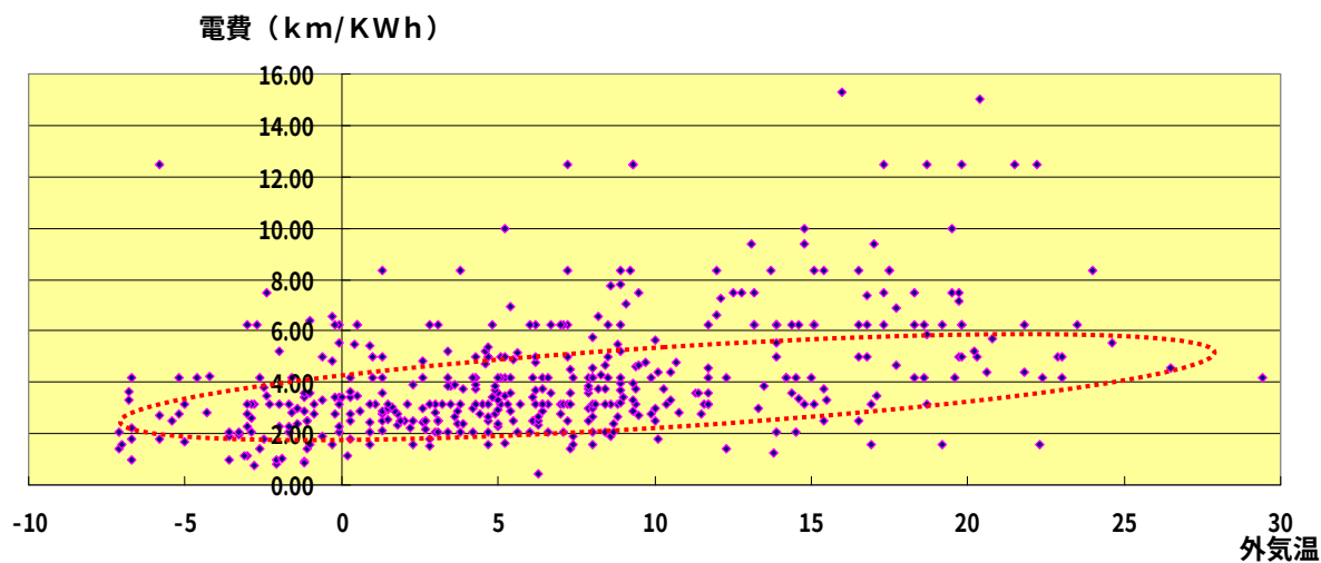
図 5.17 外気温別電費（エアコン無）
