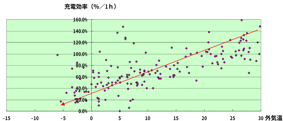
図 5.21 外気温別充電効率散布図 (急速充電)
